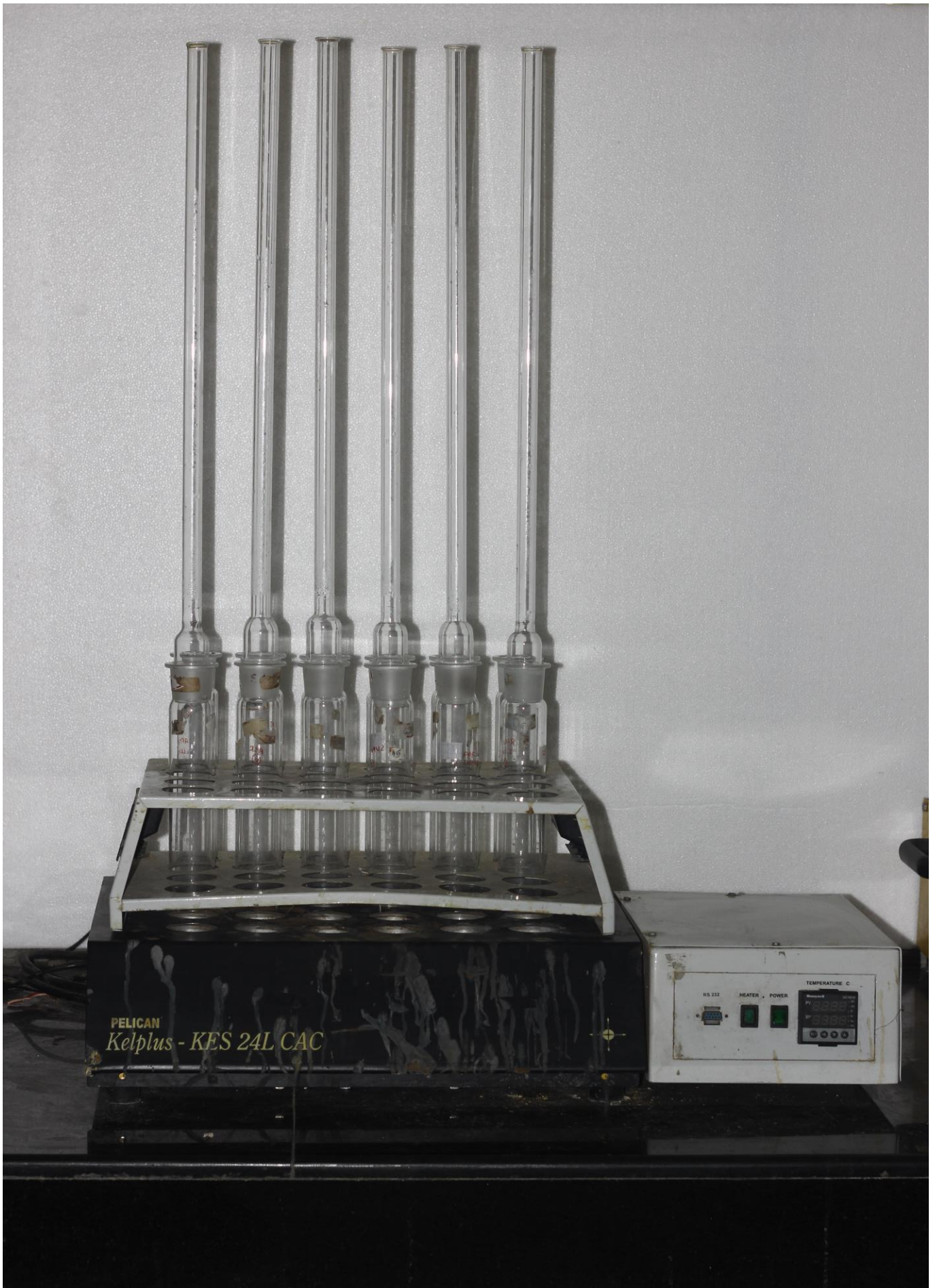
COD Digester
